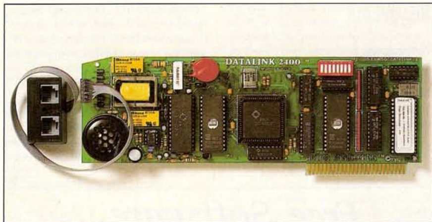
DataLink 2400
